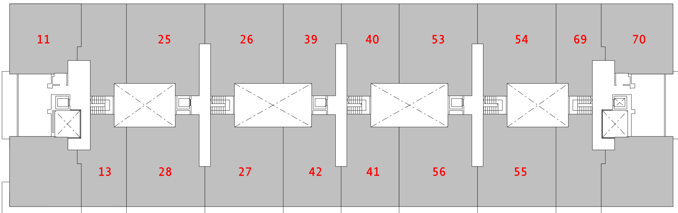
PLANTA ATICO
